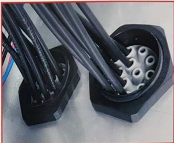
인입완료(접속함내부)
